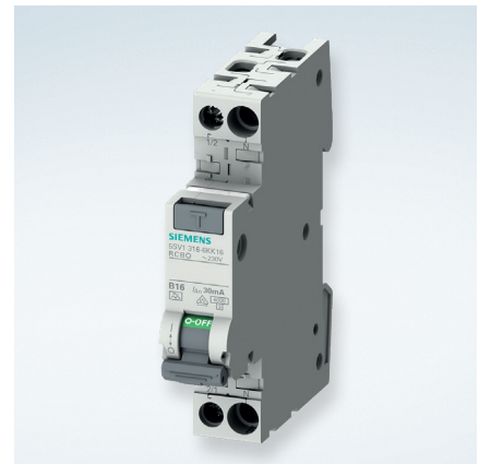
FI/LS-Schalter 5SV1 in nur 1 TE
